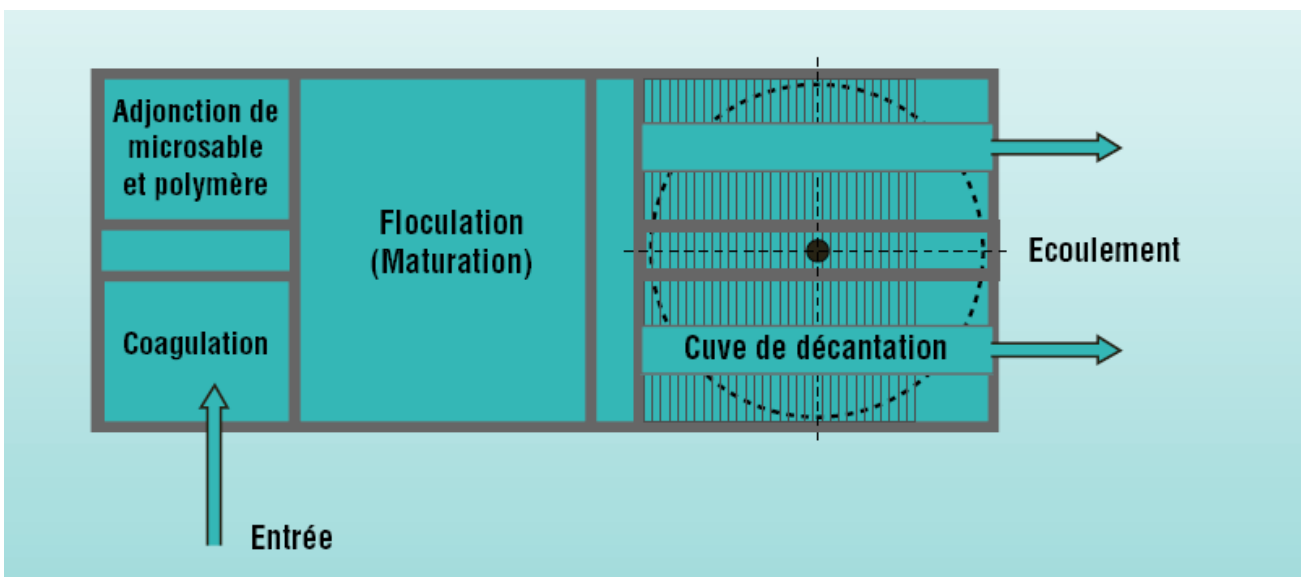
Procédé ACTIFLO® : plan de l'installation
