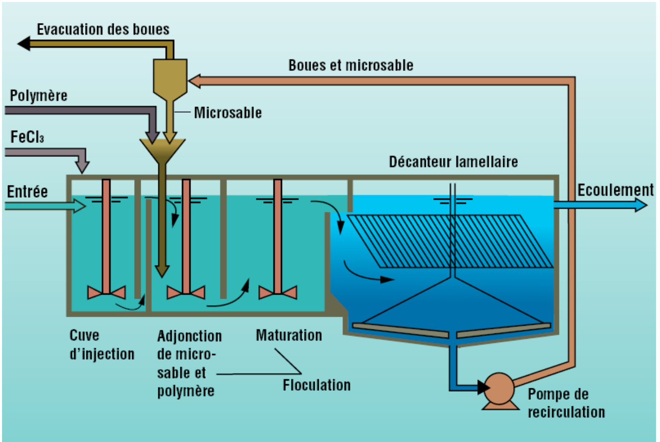
ACTIFLO® : coupe schématique longitudinale
